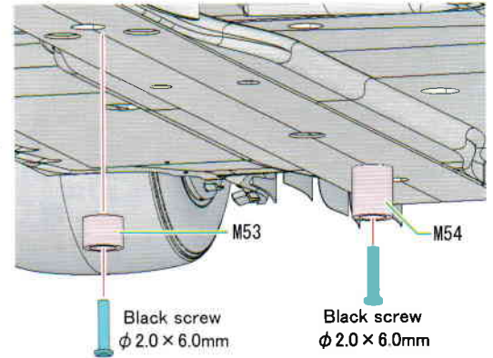
Spacer
