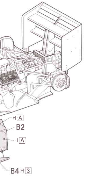
18 ラジエターダクトの取り付け Attaching radiator duct
